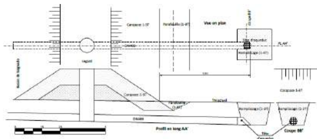
Figure 216: Vue de détail du débouché en mer de l'ouvrage hydraulique
