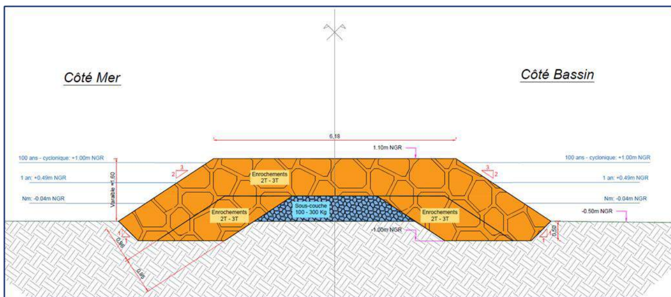
Figure 229 : Coupe type de l'enrochement – Tronçon Principal
