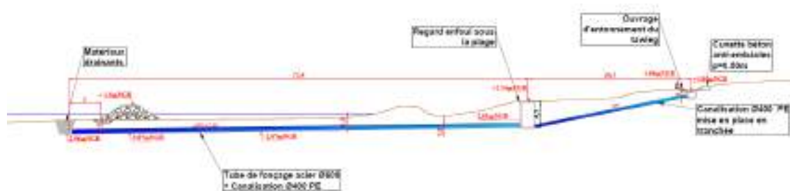
Figure 215: Principe d'implantation de la canalisation
