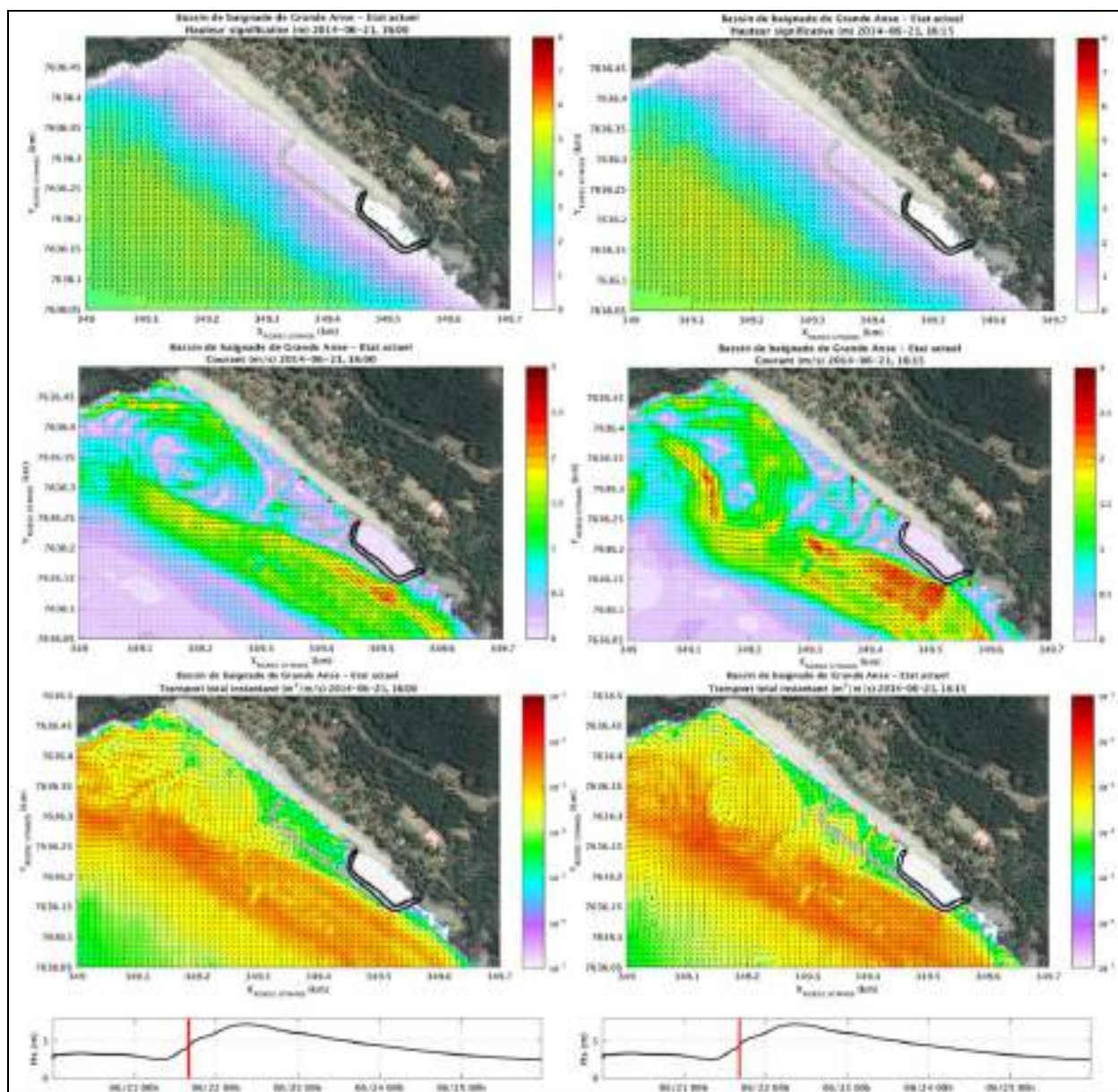
Figure 5-15 : Propagation des vagues (en haut), cartes de courant (au milieu) et capacités de transport solide (en bas) - Conditions de vagues très énergétiques de houle australe (périodes longues) induisant globalement une circulation du Sud-Est vers le Nord-Ouest de l'anse.
