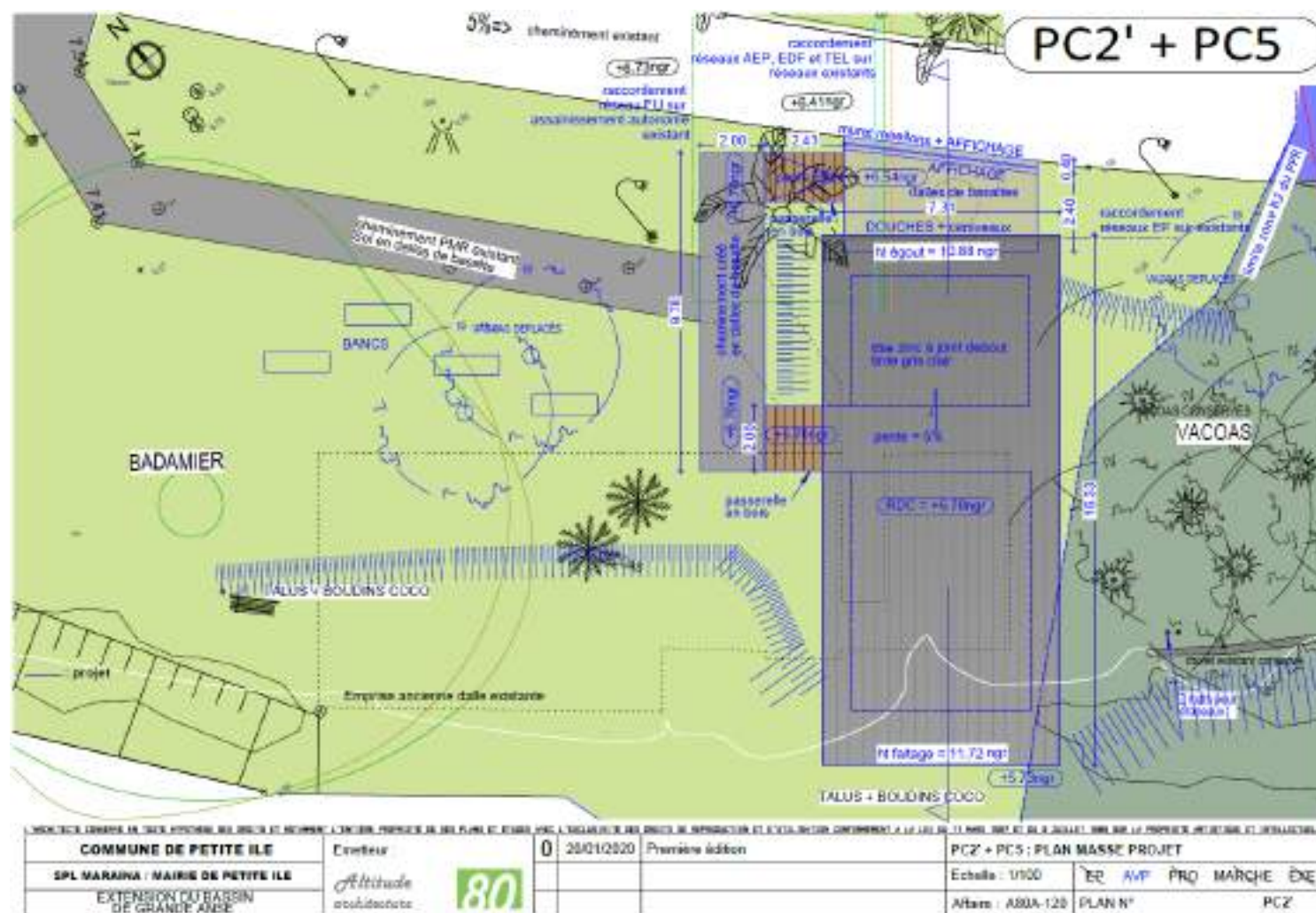
Figure 30: Plan des aménagements du poste MNS
