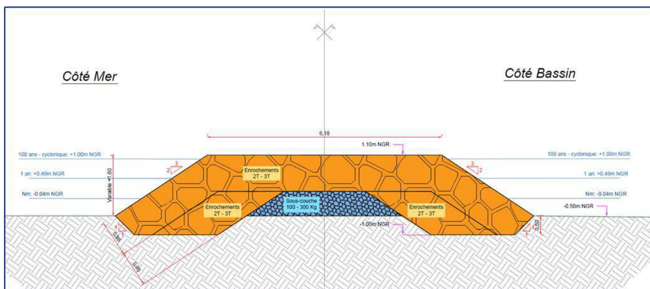
Figure 36 : Coupe type de l'enrochement – Tronçon Principal
