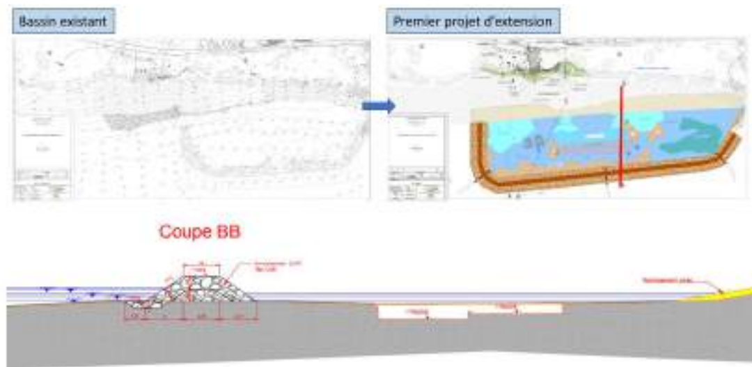
Figure 18 : Premier projet d'extension du bassin de baignade et coupe-type sélectionnée (B-B') pour la mise en place du modèle 1DH SWASH.
