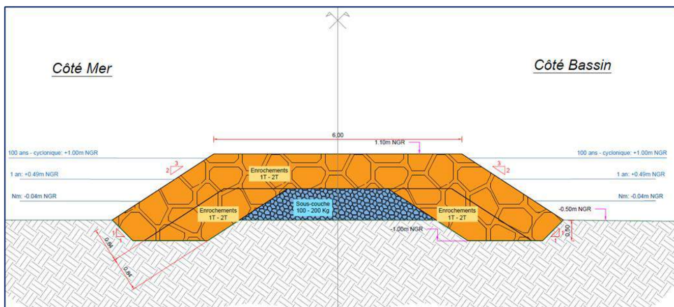
Figure 35 : Coupe type de l'enrochement – Tronçon de retour
