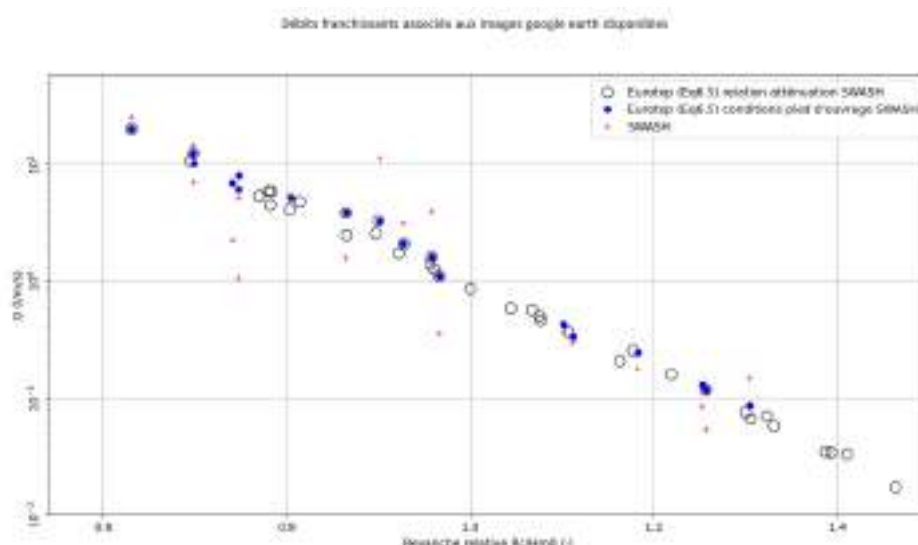
Figure 38 : Comparaison des débits franchissants (Q en l/m/s) estimés à partir de la modélisation SWASH et de la formule empirique de l'Eurotop pour les différentes images Google Earth sélectionnées entre 2015 et 2021. Les débits franchissants sont ici représentés en fonction de la revanche relative Rc/Hm0 (représentation classique).
