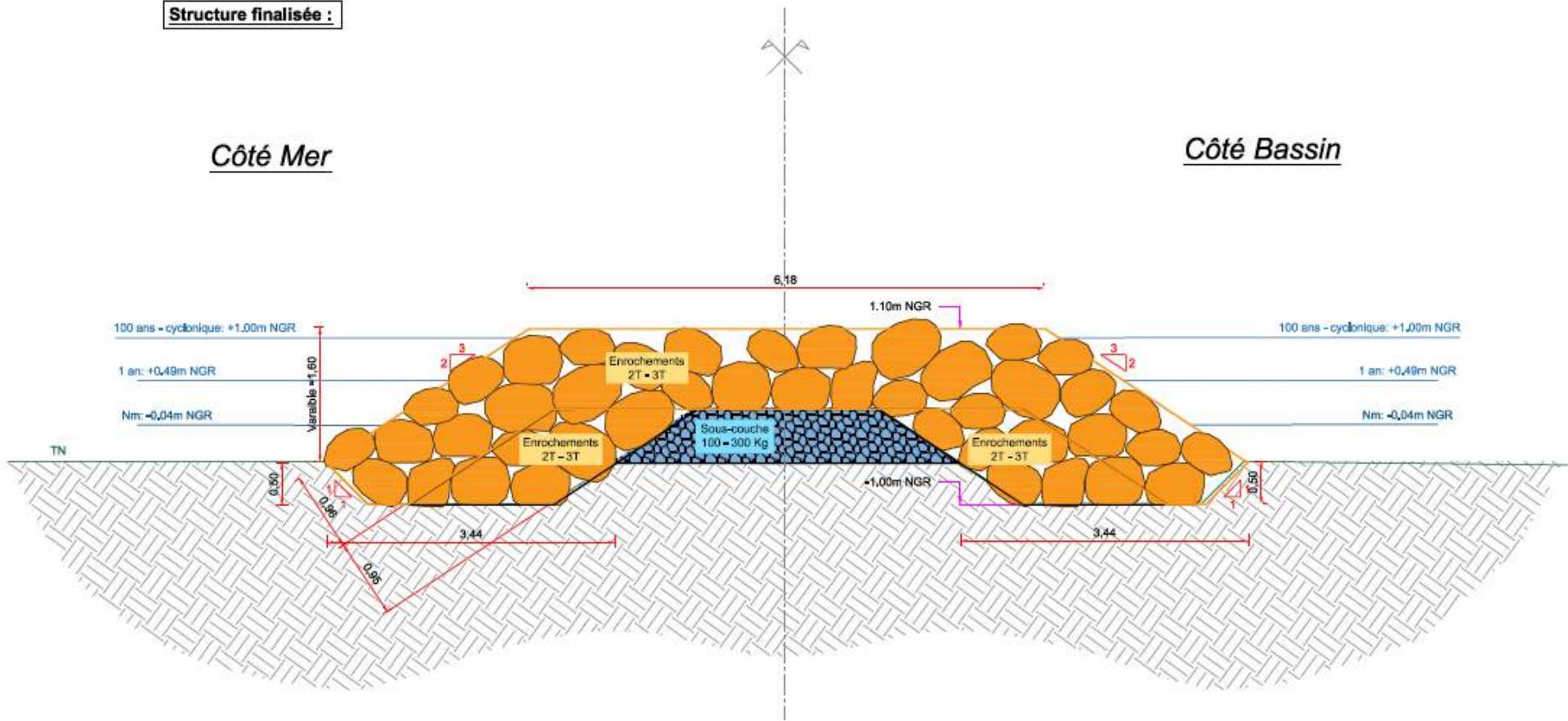
Figure 230: Plan de masse de la protection en enrochement
