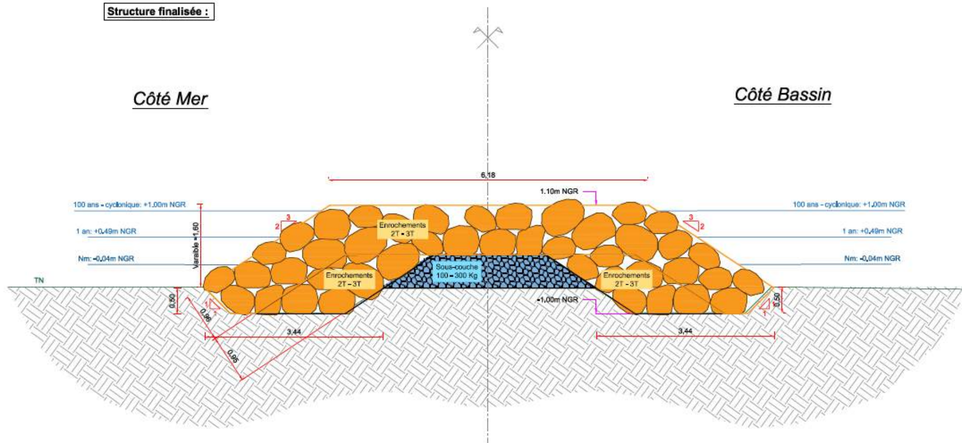
Figure 37: Plan de masse de la protection en enrochement
