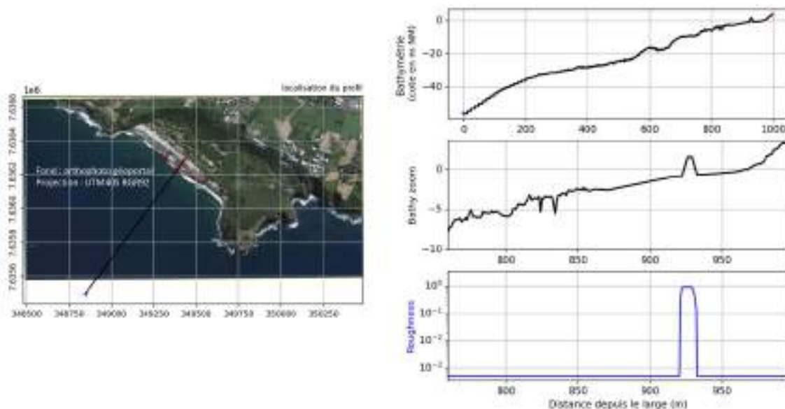
Figure 19 : Modèle 1DH SWASH mis en place pour le premier projet d'extension du bassin, avec une configuration d'ouvrage avec une arase initialement prévue à la cote +1.5 m NGR : localisation du profil, bathymétrie (en m par rapport au niveau moyen, i.e. -0.044 m NGR), et rugosité prescrite afin de tenir compte de l'effet de l'enrochement en enrochement sur les franchissements par paquets de mer.
