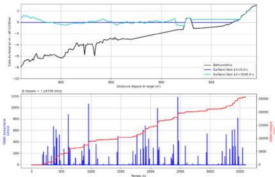
Figure 23 : Résultats du modèle SWASH (débits franchissants instantanés et intégrés au cours du temps) obtenus pour le premier projet d'extension du bassin avec une cote d'arase à +1.1 m NGR pour des conditions de vagues moyennes ( H_s=1.78 m, T_p=12.78 s) et un niveau d'eau de référence de PHMA (i.e. « 0 » sur le graphe du haut = +0.366 m NGR). Le débit franchissant moyen obtenu sur l'heure simulée est de 7.15 l/m/s.
