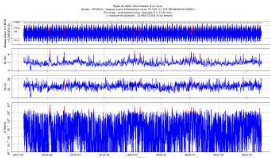
Figure 40 : Rejeu de débit franchissant (Q en l/m/s) réalisé à partir de la formule de l'Eurotop sur la période 2017-2021. Les données d'entrée de niveaux d'eau (atlas FES2014) et de vagues (Hs et Tp extraits du modèle MARC IFREMER) sont également présentées. Les périodes représentées en rouge sont associées à des débits franchissants supérieurs au seuil sécuritaire de 10 l/m/s.
