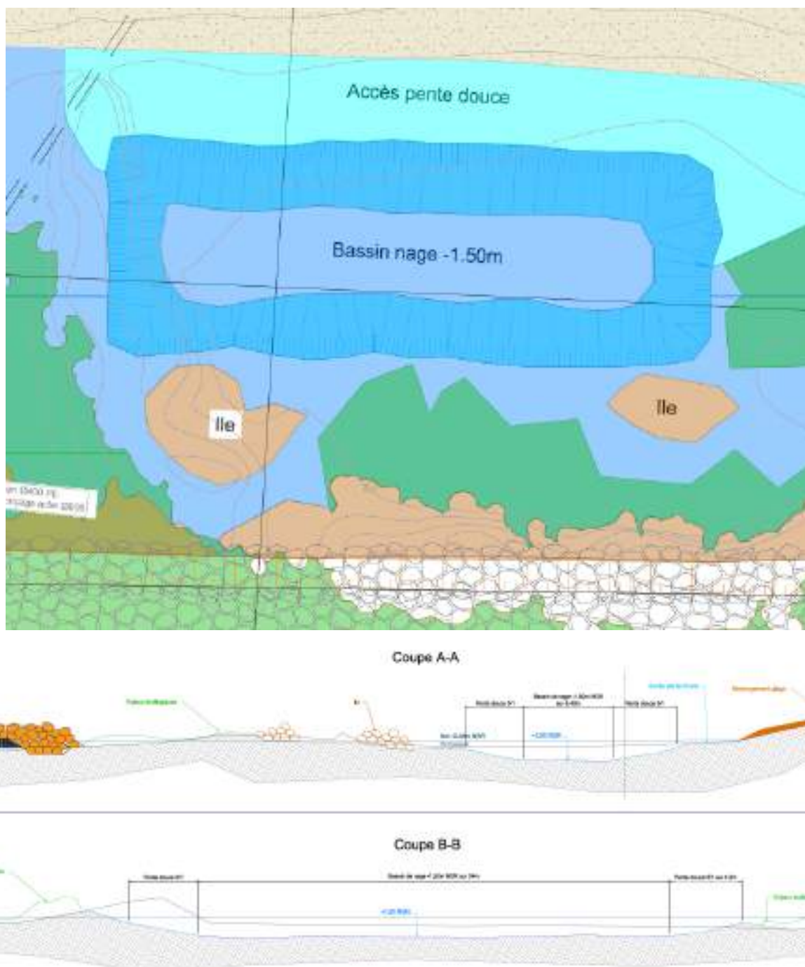
Figure 39 – Vue en plan + coupe de la fosse d'apprentissage
