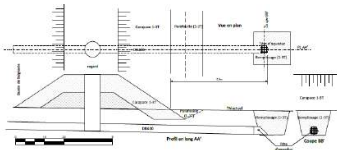
Figure 43: Vue de détail du débouché en mer de l'ouvrage hydraulique
