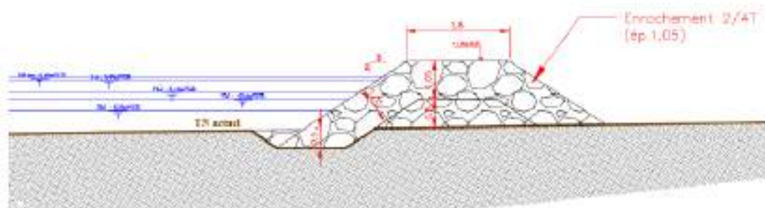
Figure 17: Coupe type de l'enrochement de protection
