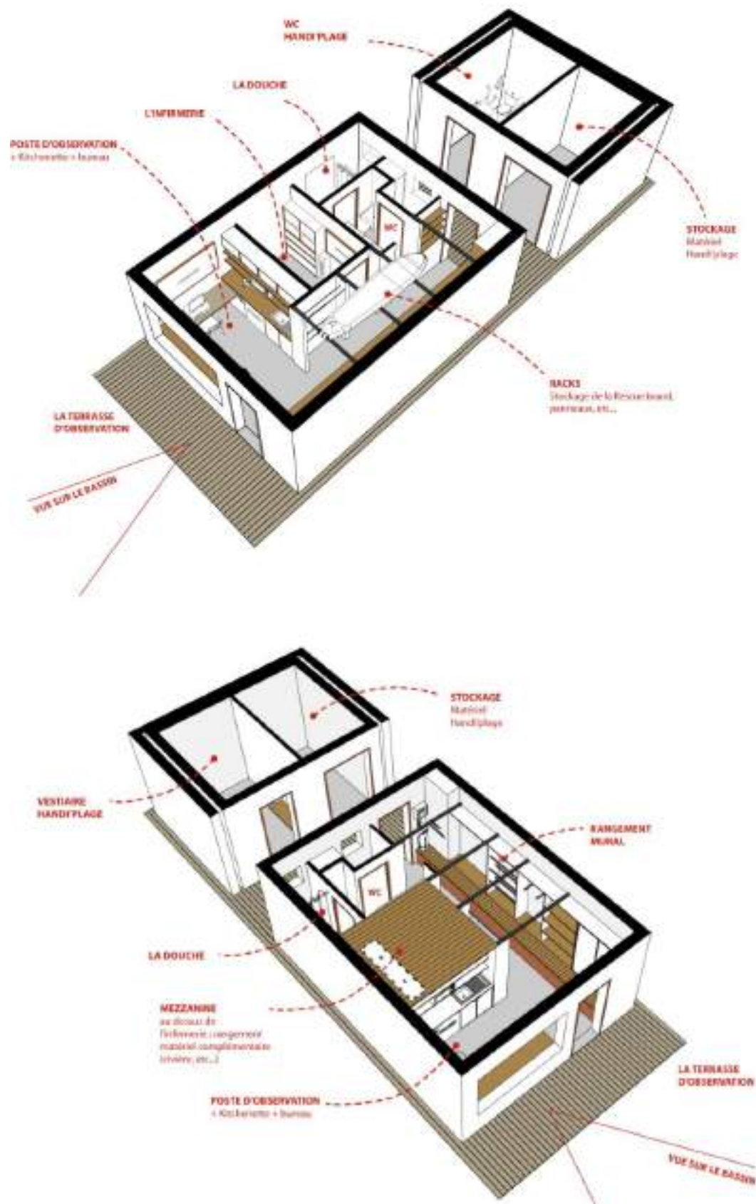
Figure 34: Vues de détails de l'organisation du poste de surveillance
