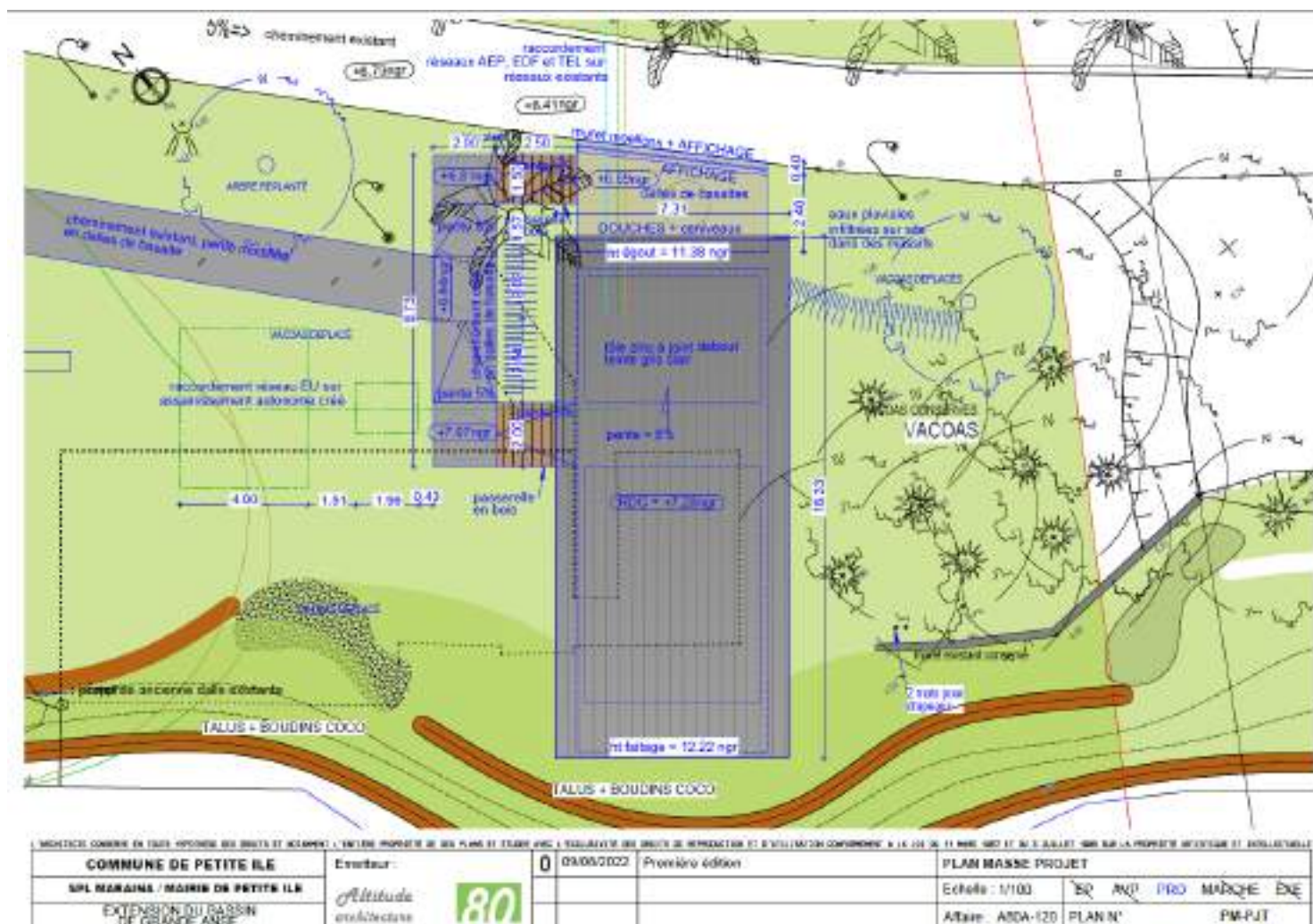
Figure 33: Plan d'implantation général du local du surveillance
