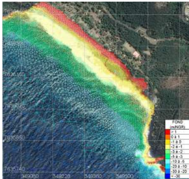
Figure 4-3 : Zoom sur la plage de Grande Anse pour le maillage et bathymétrie de la modélisation numérique des états de mer. Les cotes du fond sont exprimées en mètre par rapport à l'IGN 89. Projection RGR92 UTM40S.
