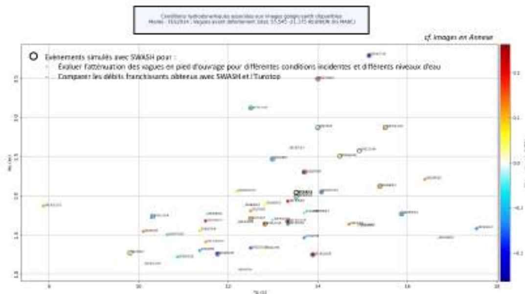
Figure 32 : Images Google Earth exploitées entre 2015 et 2021, et conditions de vagues (Hs, Tp) et de niveaux d'eau déterminées en évaluant l'heure de chaque prise de vue à partir de l'orientation des ombres à terre. Les événements entourés en noir ont été simulés avec le modèle SWASH.
