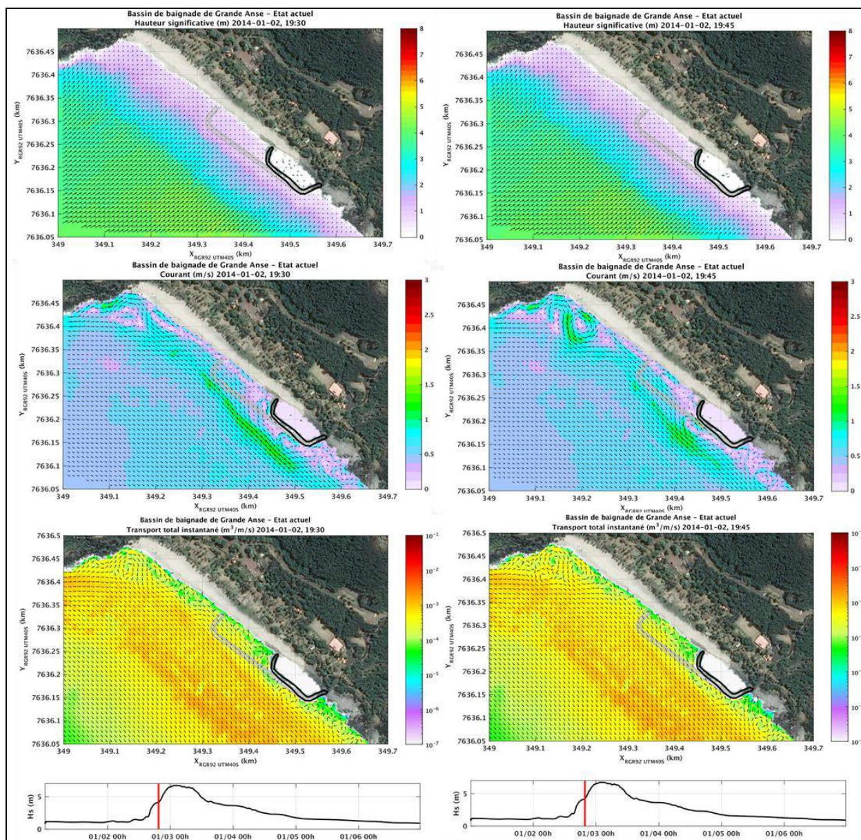
Figure 5-16 : Propagation des vagues (en haut), cartes de courant (au milieu) et capacités de transport solide (en bas) - Conditions de vagues très énergétiques de type cycloniques (périodes plutôt courtes) induisant globalement une circulation du Nord-Ouest vers le Sud-Est de l'anse.
